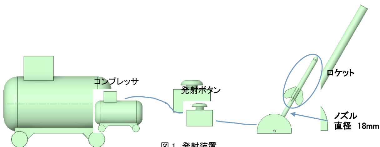
図1 発射装置
